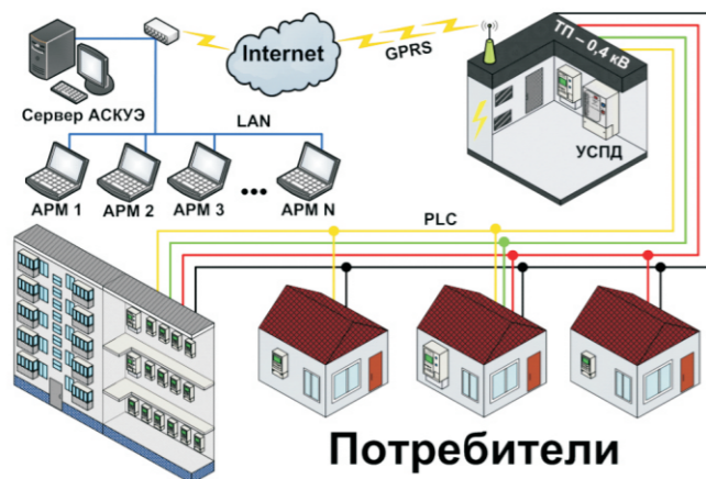
Схема передачи данных в АСКУЭ с применением технологии PLC
